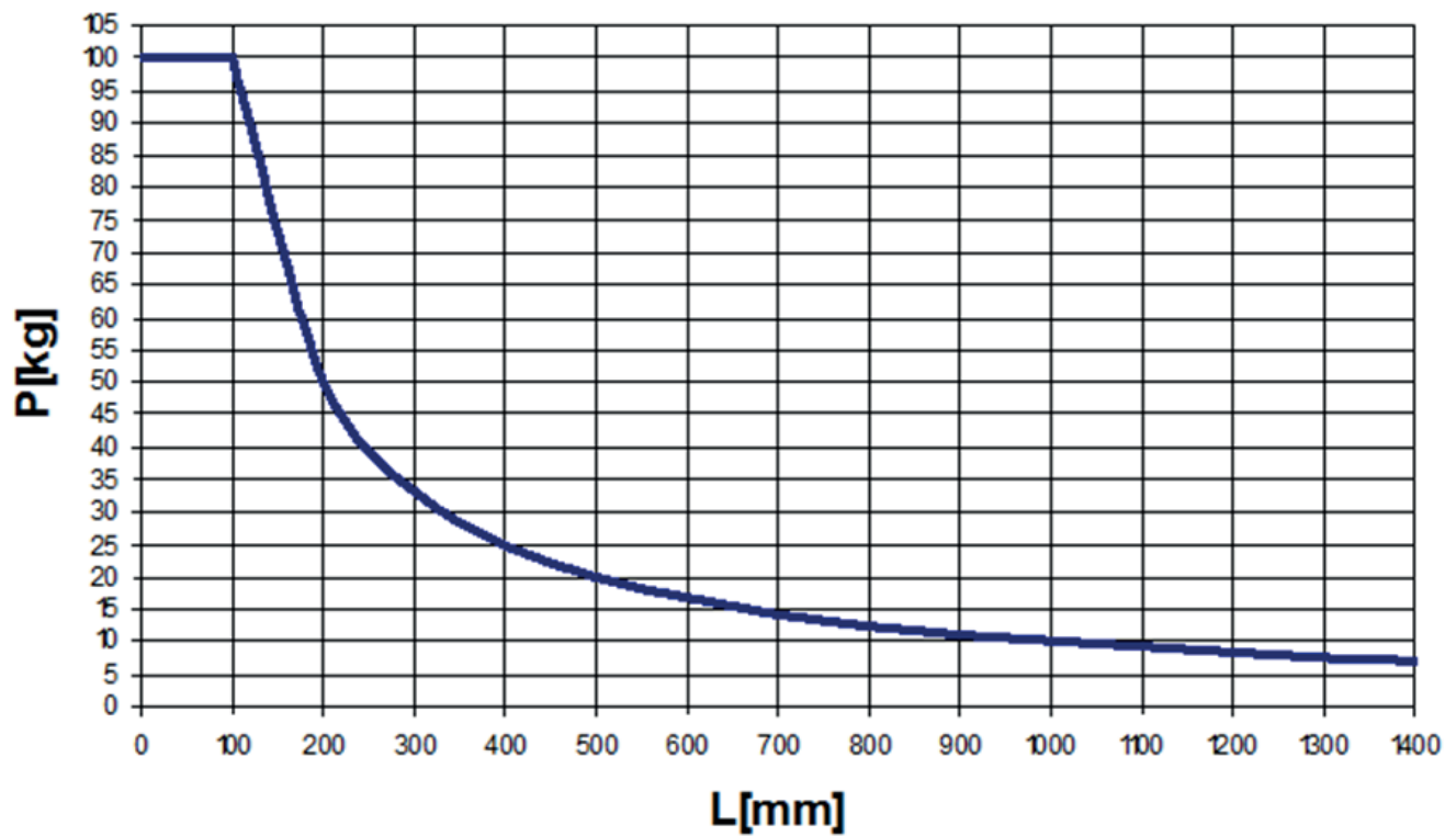
Verticaal draagvermogen t.o.v. lengte van het werkstuk (symmetrisch)
